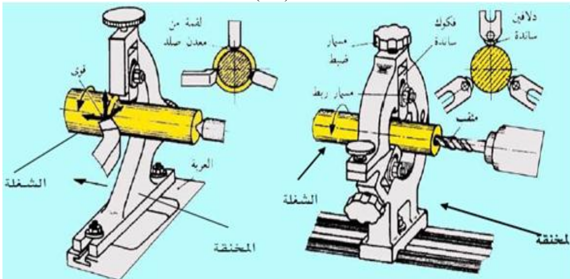
2. المخنقة المتحركة
