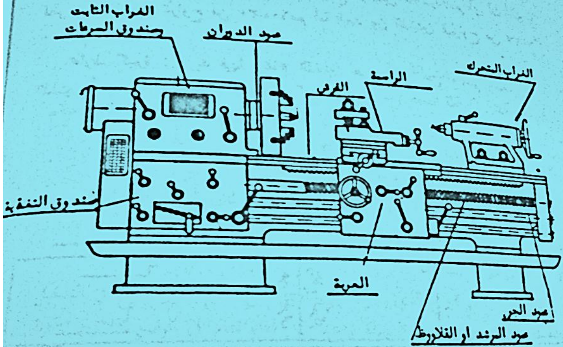
شكل (3-6) مخطط يوضح الاجزاء الرئيسية للمخرطة
